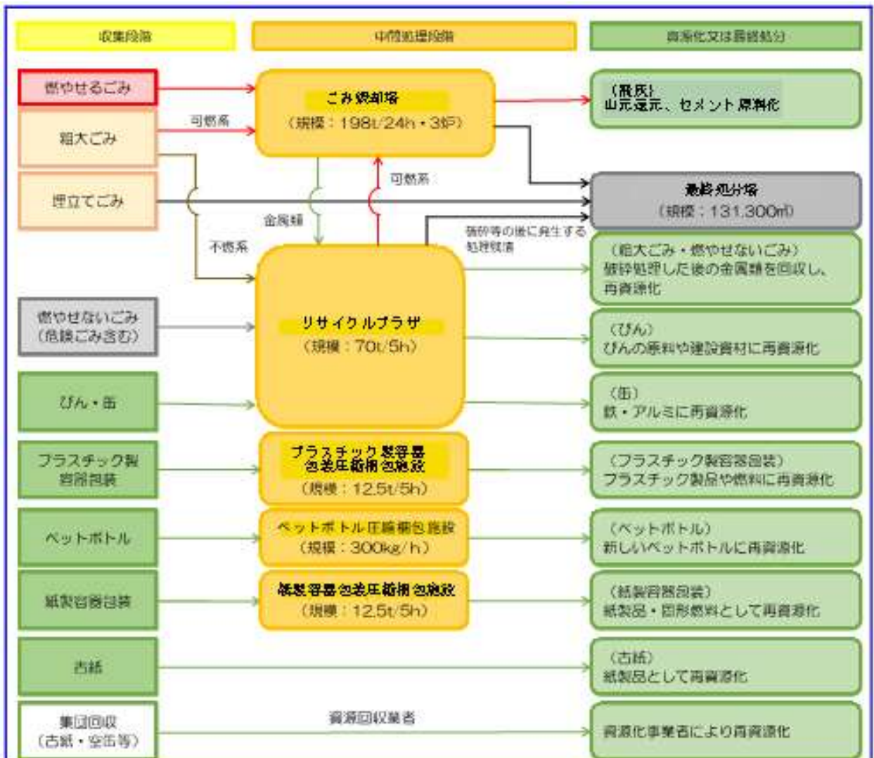
◆図表2-4 ごみ処理フロー
