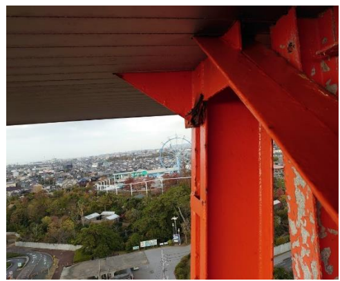
【鉄塔 展望台 下側】 腐食劣化
