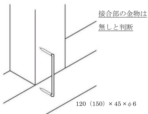
図Ⅱ.2.2.4 かすがいの例
