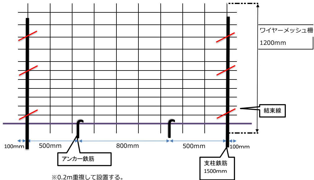
宇部市 ワイヤーメッシュ柵イメージ図
