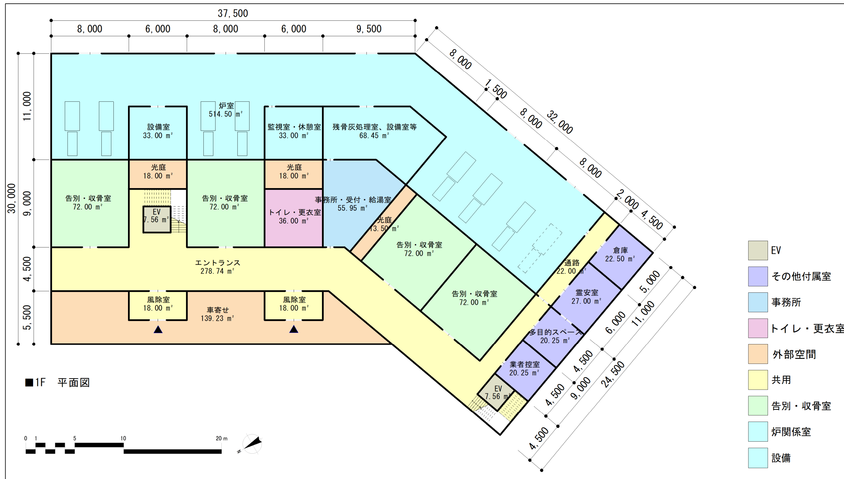
図 6-3 モデルプラン (1階)
