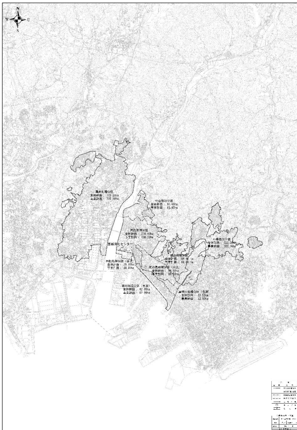
別紙 5-2 宇部市下水道処理区域一般平面図（西部処理区拡大）
