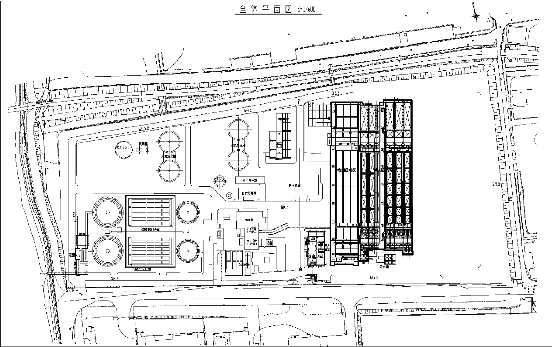
別紙 4 西部浄化センター一般平面図
