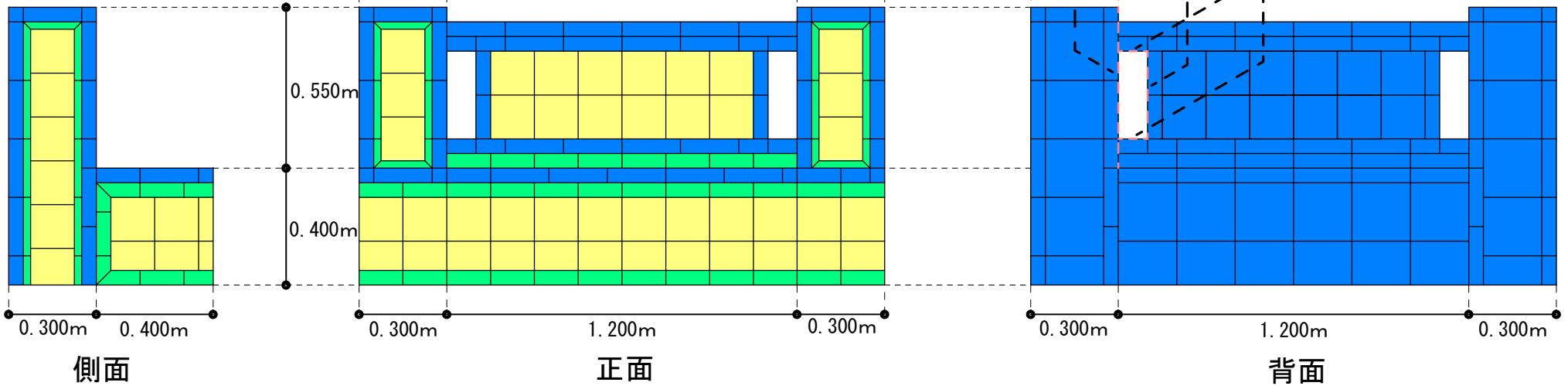
【立面図】
