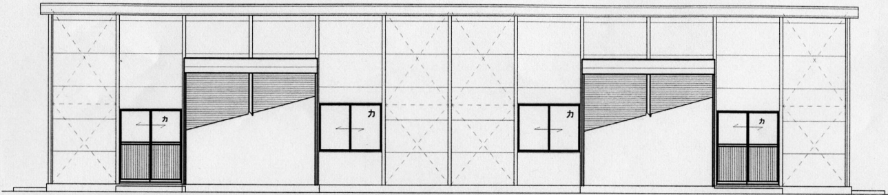
Y0 立面図
