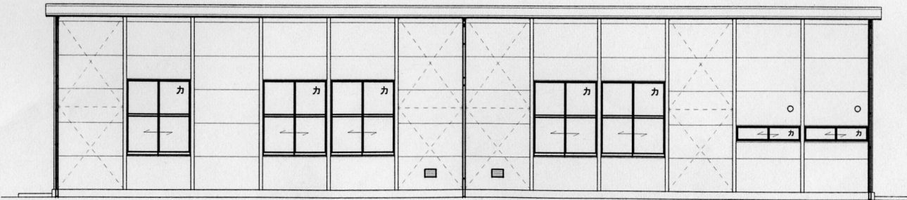
Y5 立面図
