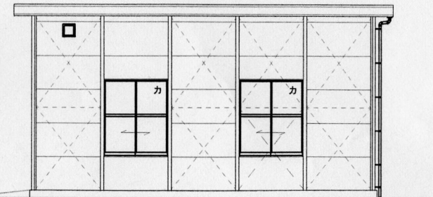
X12 立面図
