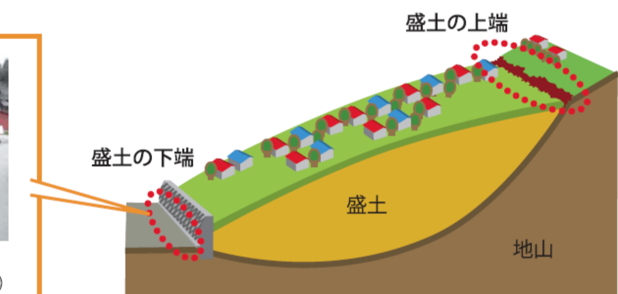
擁壁下端のハラミ出し (提供：社団法人 全国宅地擁壁技術協会)
