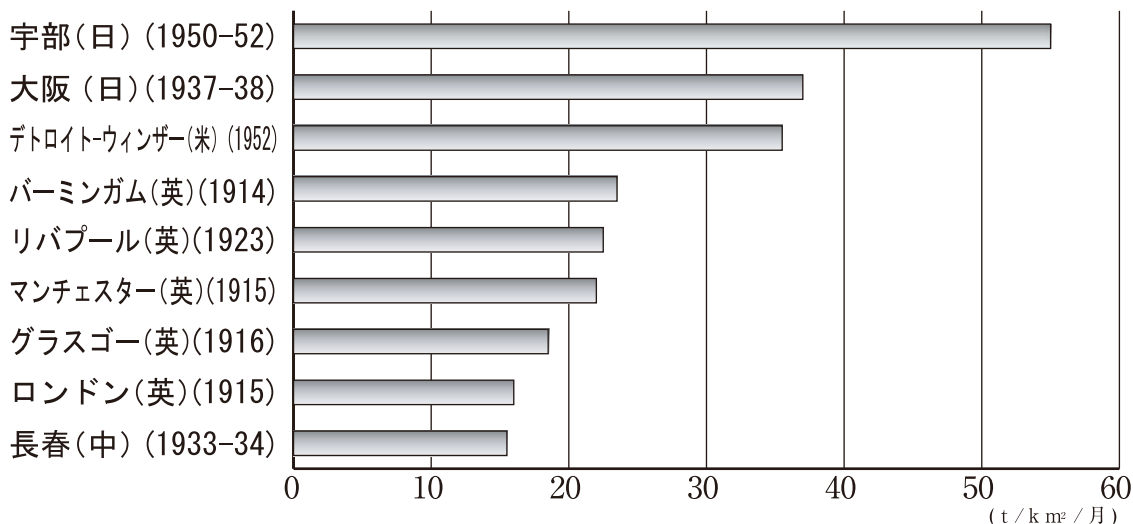
宇部市で降下煤塵を測定開始した当時の国内外諸都市の煤塵量
