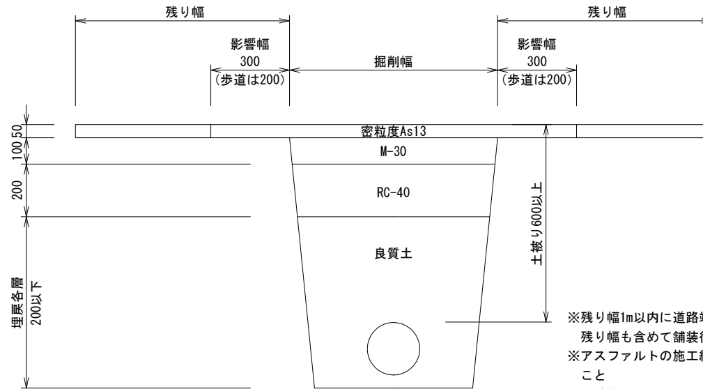
復旧断面図
