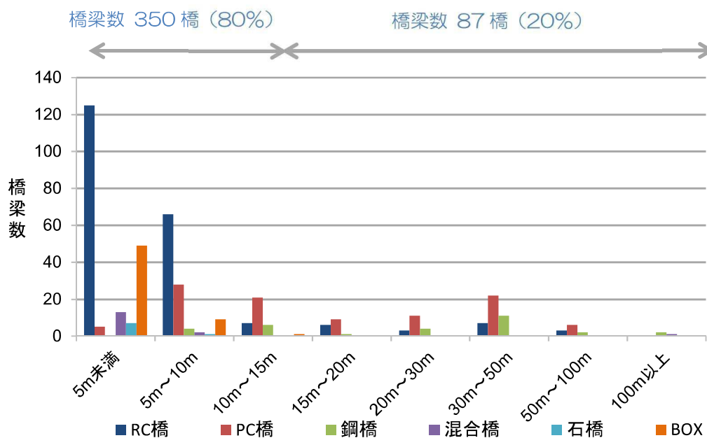
図-2.3 橋長・橋種ごとの橋梁数
