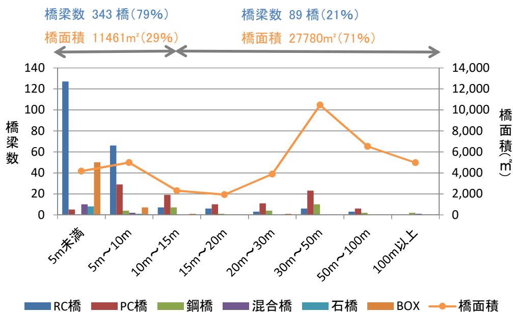
図-2.3 橋長・橋種ごとの橋梁数及び橋面積
