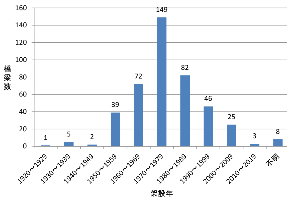
図-2.4 架設年別の橋梁数
