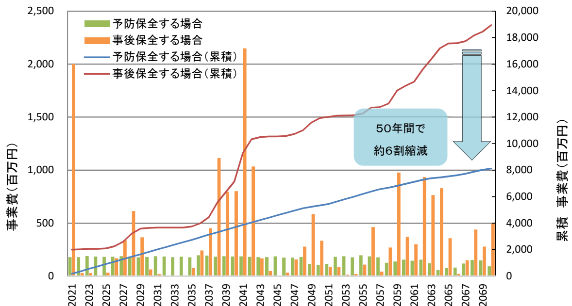
図-6.2 長寿命化 修繕計画対象橋梁全体のコスト縮減効果
