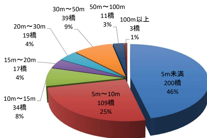
図-2.2 橋長ごとの橋梁数
