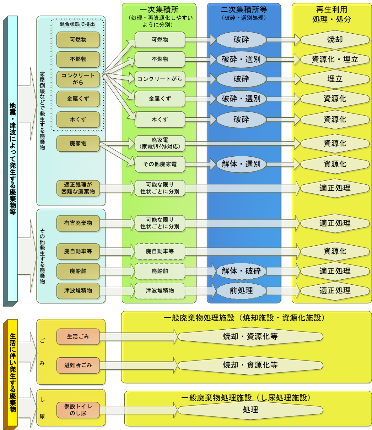
図表 4-6 災害廃棄物等の処理の流れ
