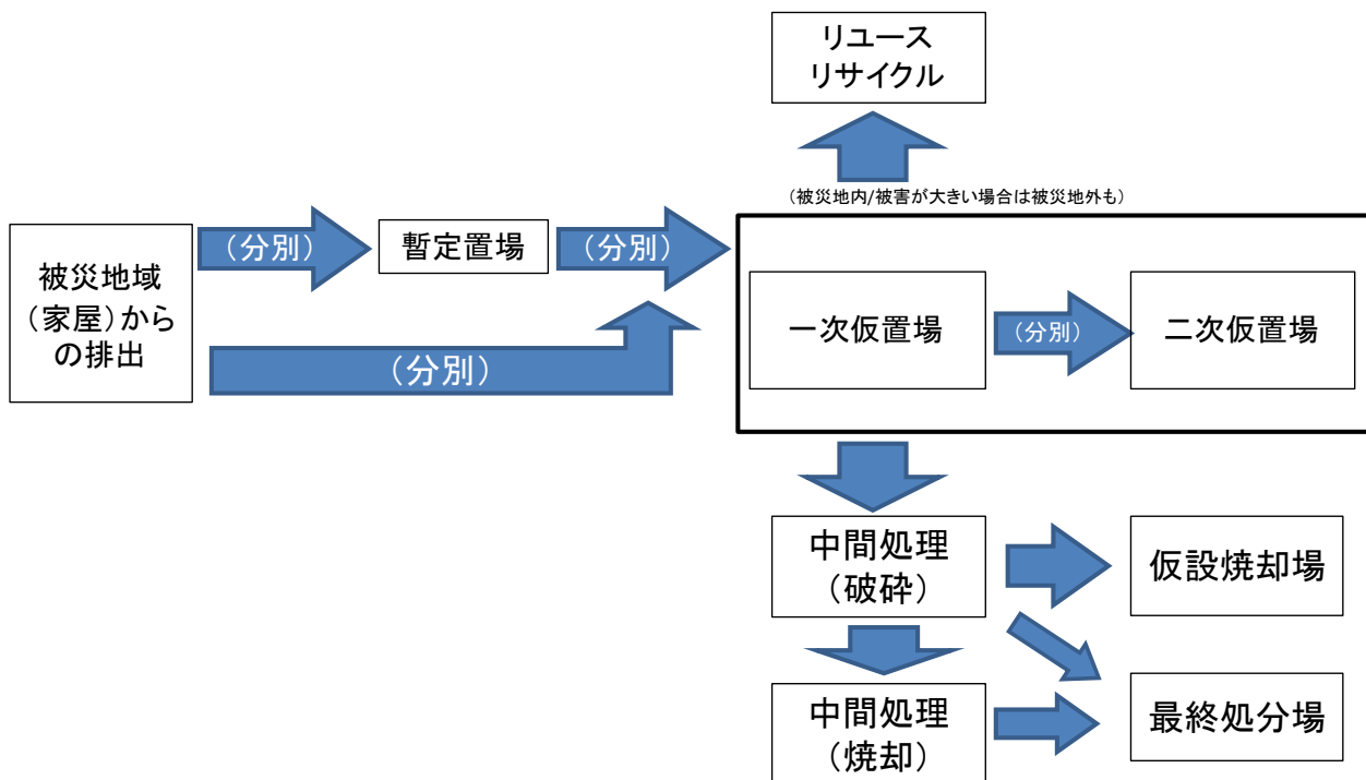
図表 4-2-2 基本的な災害廃棄物の分別・処理フロー
