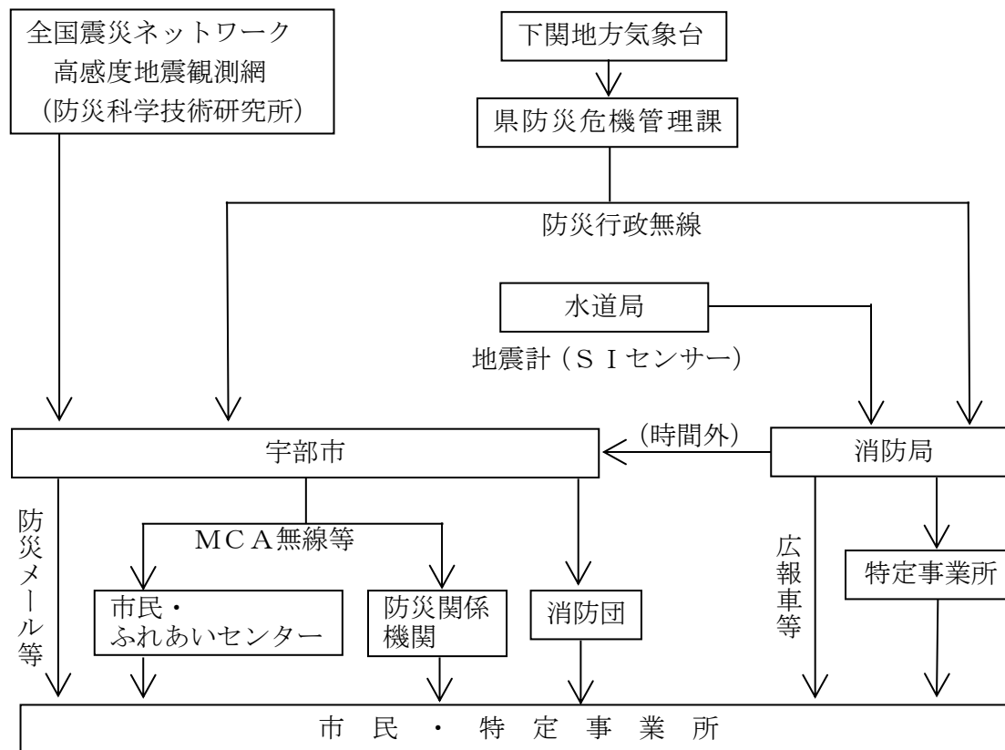
伝達系統図
